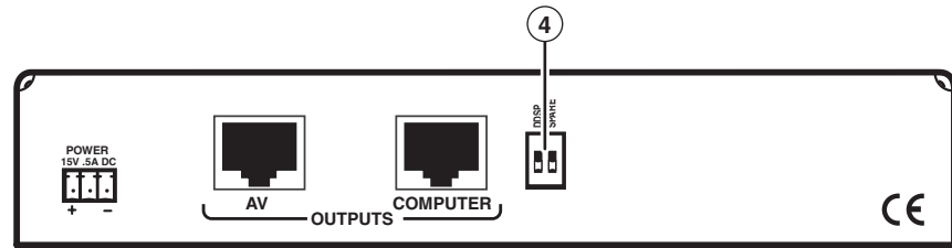
TP T 15HD AV rear panel control
