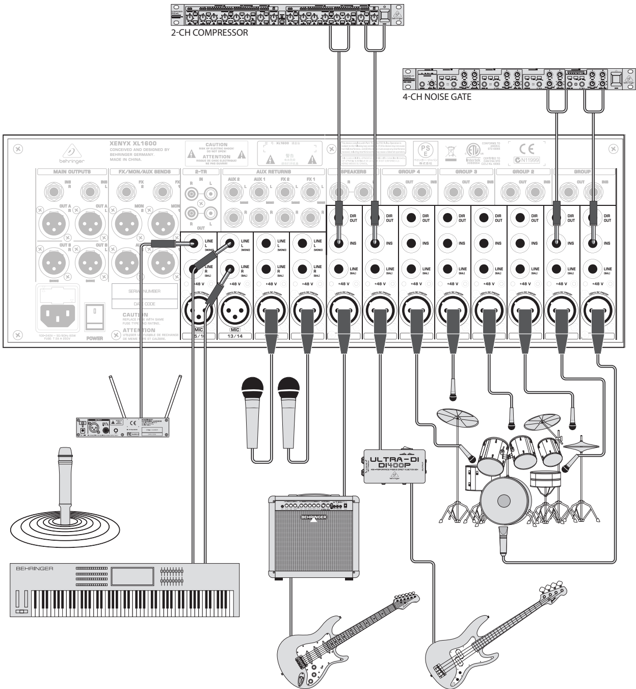
Fig. 2.1: Input wiring
