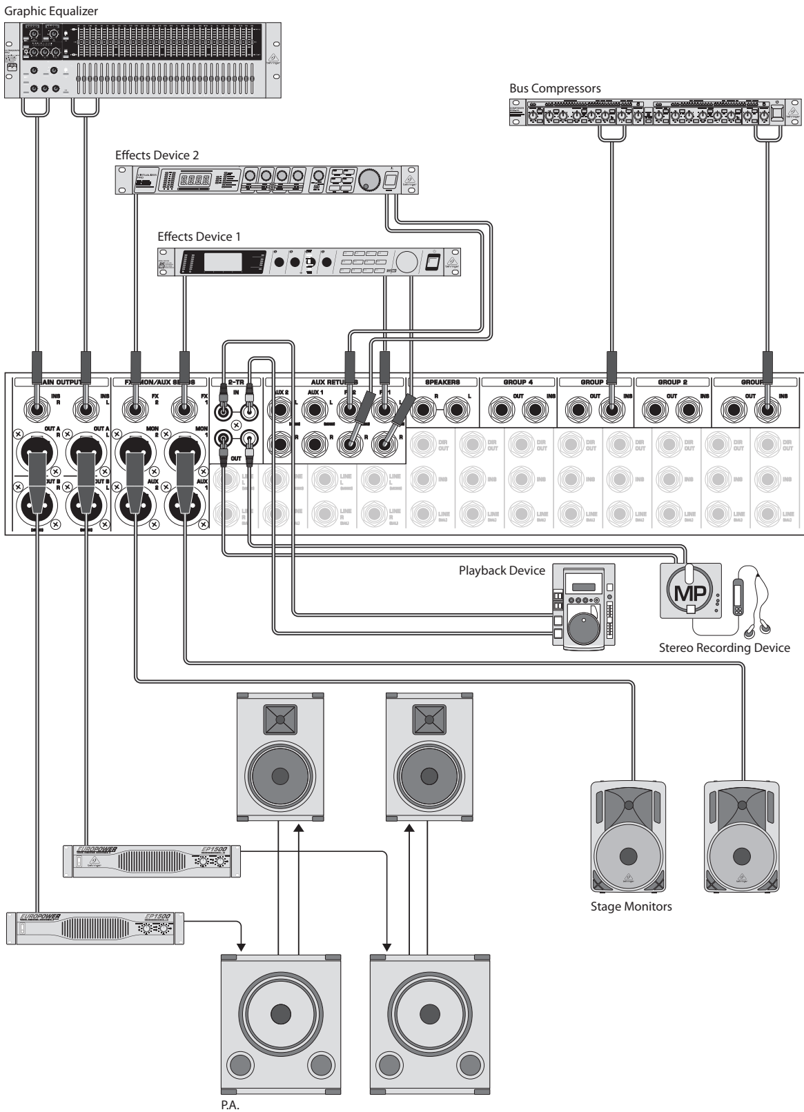
Fig. 2.2: Output wiring
